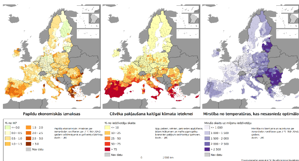
karte 7 Klimata pārmaiņu ietekme NUTS 3. līmeņa reģionos pie zemeslodes sasīšanas par 2 °C līdz 2050. gadam
