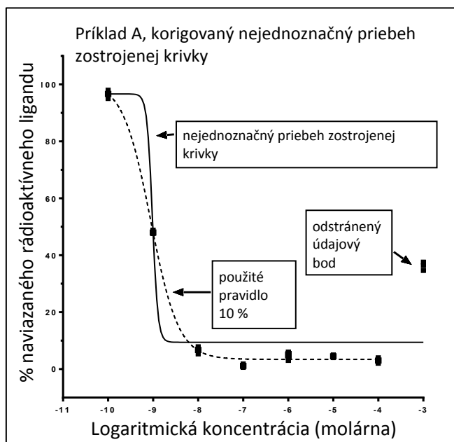
Obrázok 2: Príklady, krivky kompetitívnej väzby pri použití a bez použitia pravidla 10 %.
