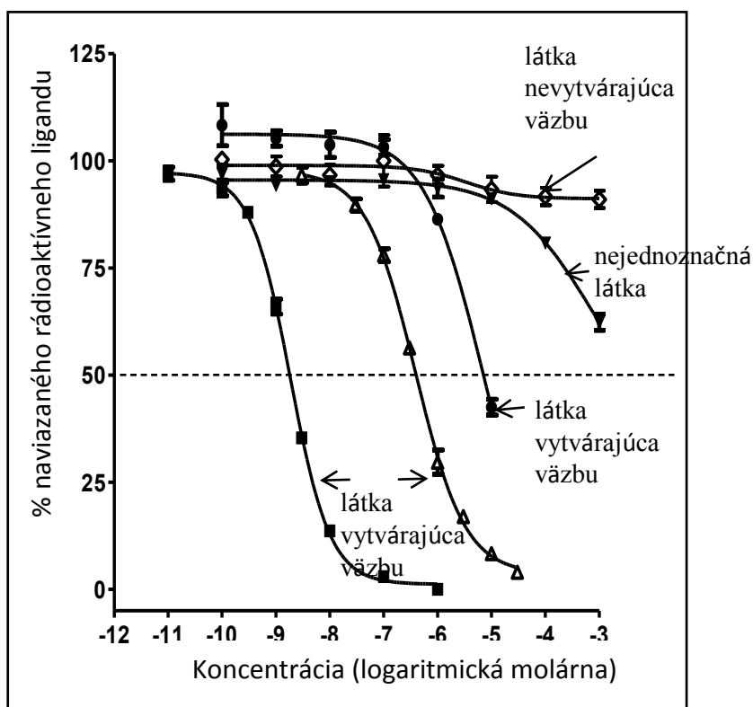
Obrázok 1: Príklady klasifikácie testovanej chemikálie pomocou krivky kompetitívnej väzby.
