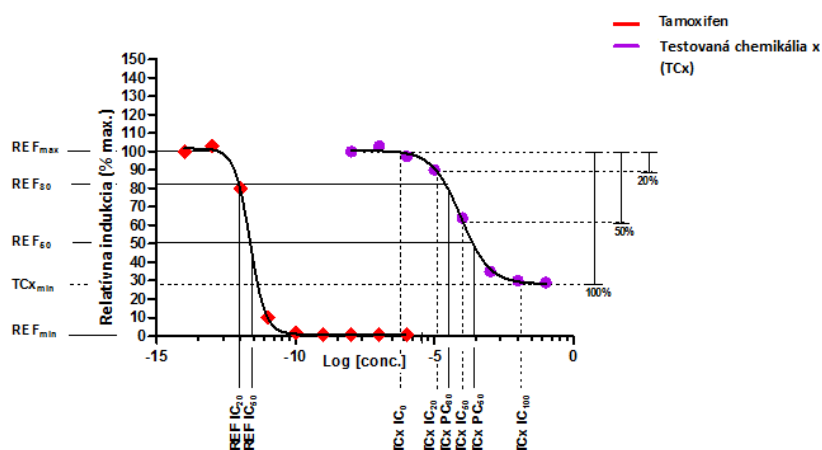
Obrázok 4: Prehľad parametrov určených v skúške antagonistu
