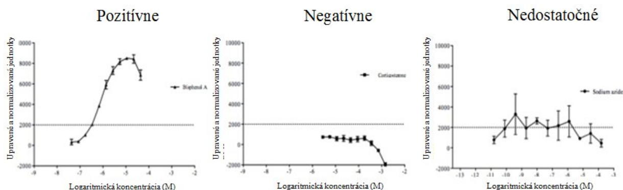
Obrázok 5: Príklady agonistu: pozitívne, negatívne a nedostatočné údaje
