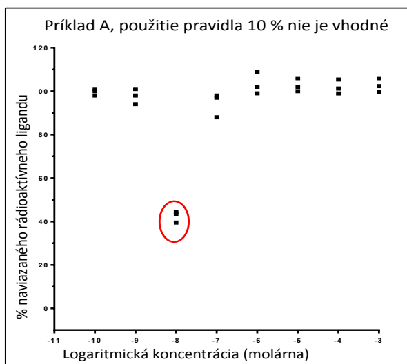
Obrázok 3: Príklady, údaje kompetitívnej väzby, pri ktorých nie je vhodné použiť pravidlo 10 %.
