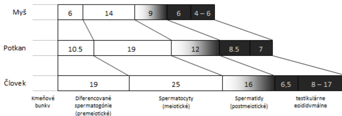
Obr. 1: Porovnanie obdobia vývoja (v dňoch) samčej zárodočnej bunky u myší, potkanov a ľudí. V časových úsekoch, ktoré sú vytieňované, nedochádza k oprave DNA.
