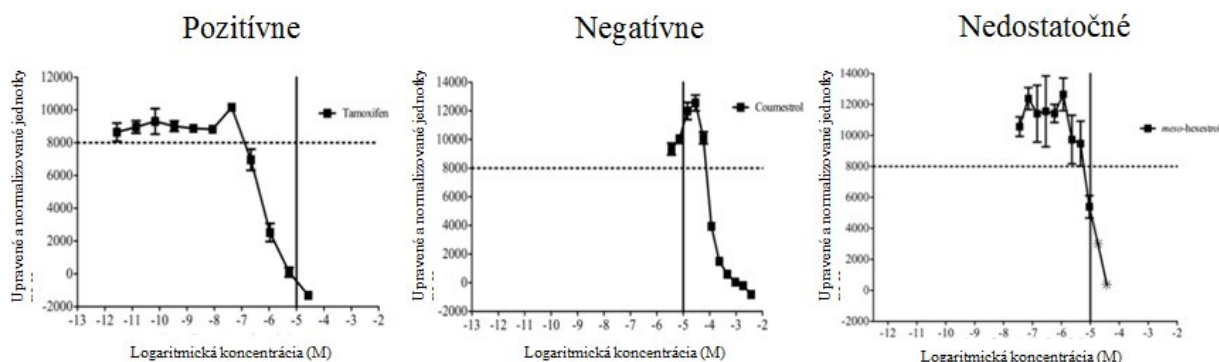
Obrázok 6: Príklady antagonistu: pozitívne, negatívne a nedostatočné údaje
