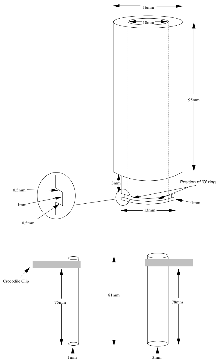
FIGURA 2: DIMENSIUNILE TUBULUI DE POLITETRAFLUORETILENĂ (PTFE) ȘI A TUBURILOR RECEPTORE ȘI A ELECTROZILOR UTILIZAȚI
