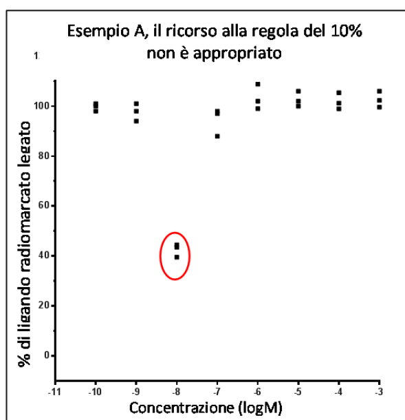
Grafico 3. Esempi di curve di legame competitivo in cui non è appropriato applicare la regola del 10 %.
