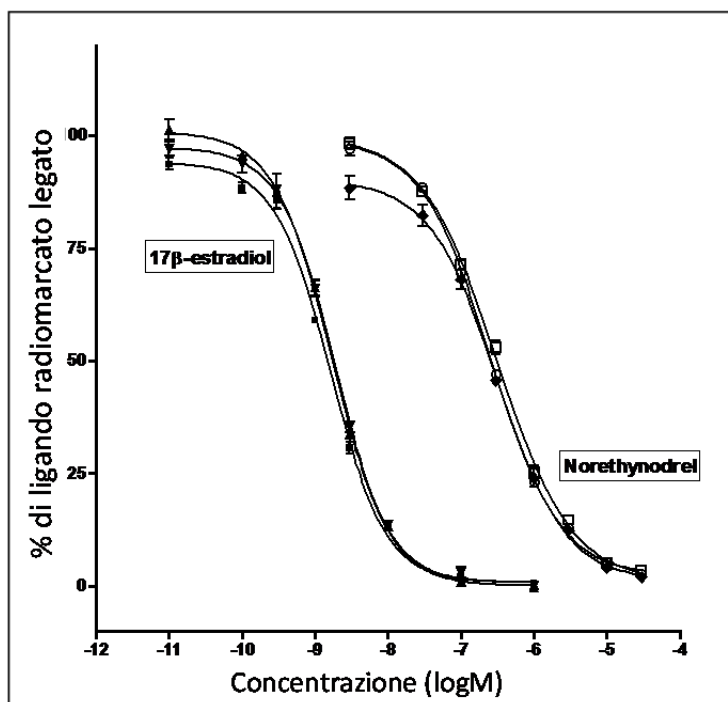
Grafico 1. Esempi di curve di legame competitivo per la sostanza estrogenica di riferimento e il ligando debole di controllo.
