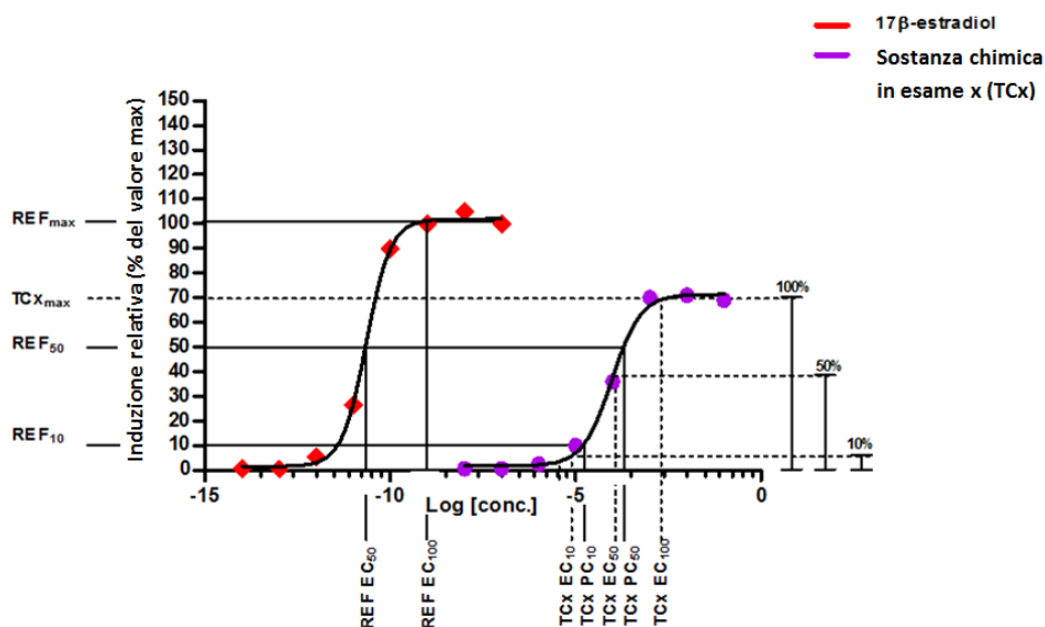
Grafico 3: Parametri determinati nella prova sull'effetto agonista
