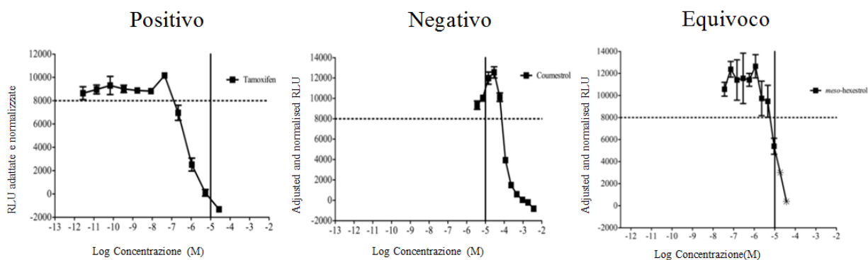
Grafico 6: Esempi di risultati positivi, negativi e equivoci per l'effetto antagonista
