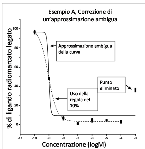
Grafico 2. Esempi di curve di legame competitivo con e senza applicazione della regola del 10 %.
