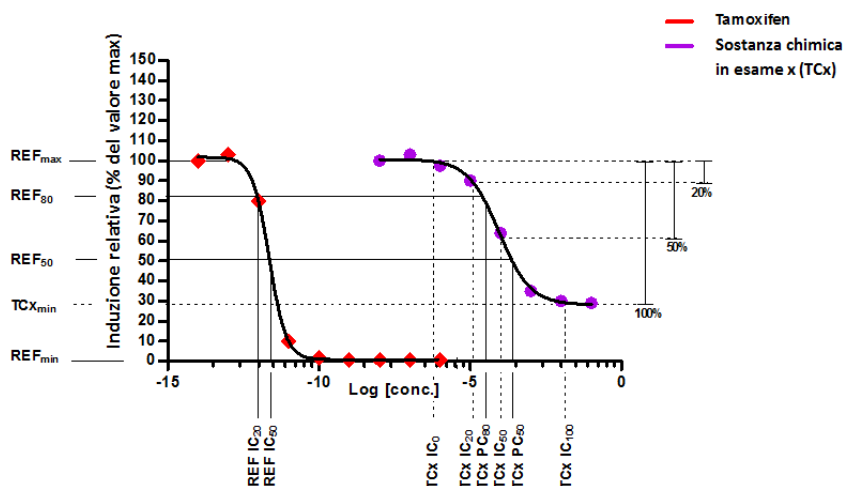
Grafico 4: Parametri determinati nella prova sull'effetto antagonista
