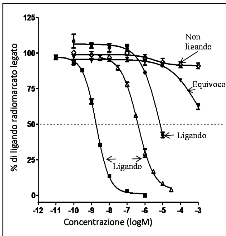
Grafico 1: Esempi di classificazione della sostanza chimica in esame in base ad una curva di legame competitivo.
