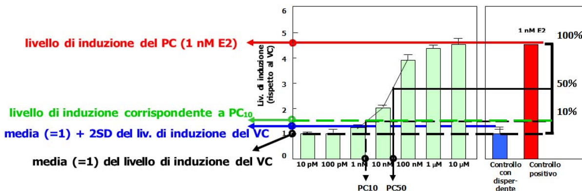
Grafico 1: Esempio di deduzione dei valori relativi al PC. Il PC (1 nM di E2) è incluso in ciascuna piastra di prova
