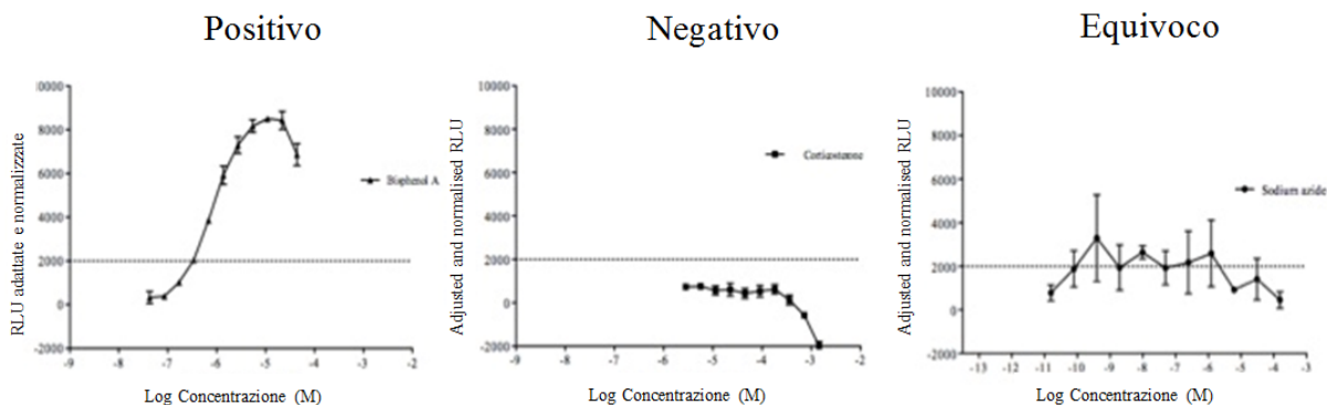
Grafico 5: Esempi di risultati positivi, negativi e equivoci per l'effetto agonista
