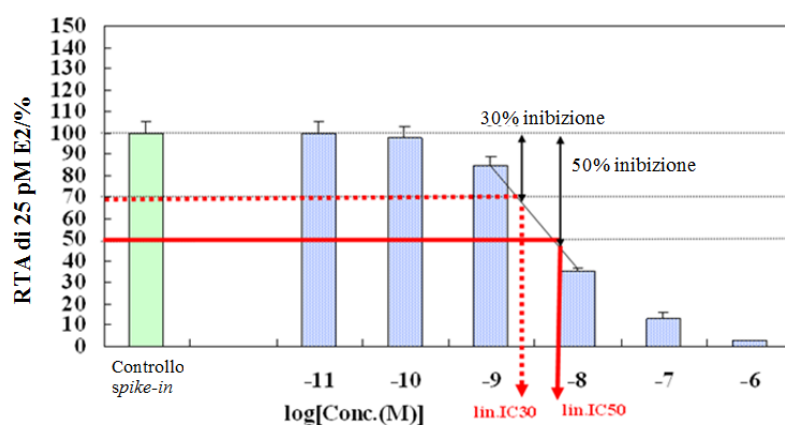
Grafico 2: Esempio di deduzione dei valori relativi all'IC. Il controllo spike-in (25 pM di E2) è incluso in ciascuna piastra di prova
