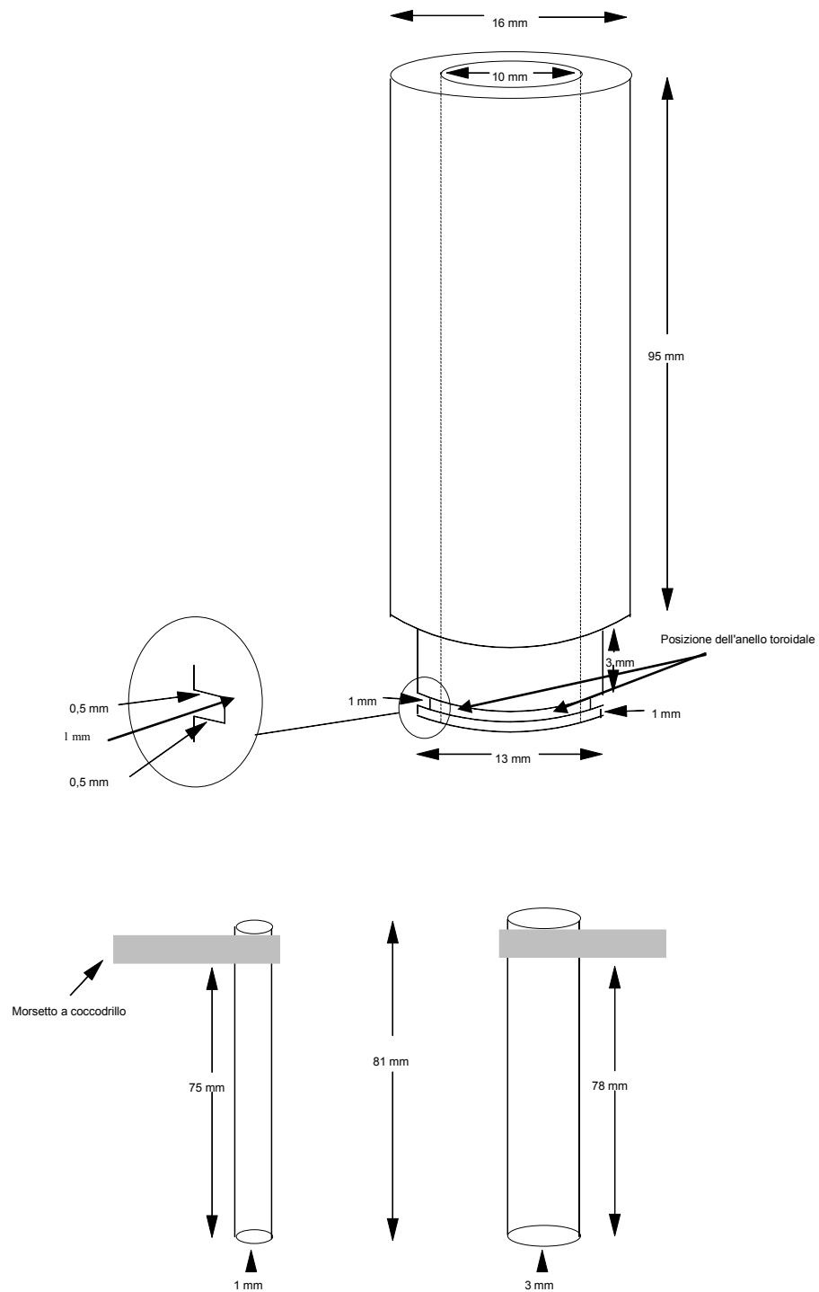
FIGURA 2: DIMENSIONI DEL TUBO IN POLIETRAFLUOROETILENE (PTFE), DEL CILINDRO CONTENITORE E DEGLI ELETTRODI UTILIZZATI
