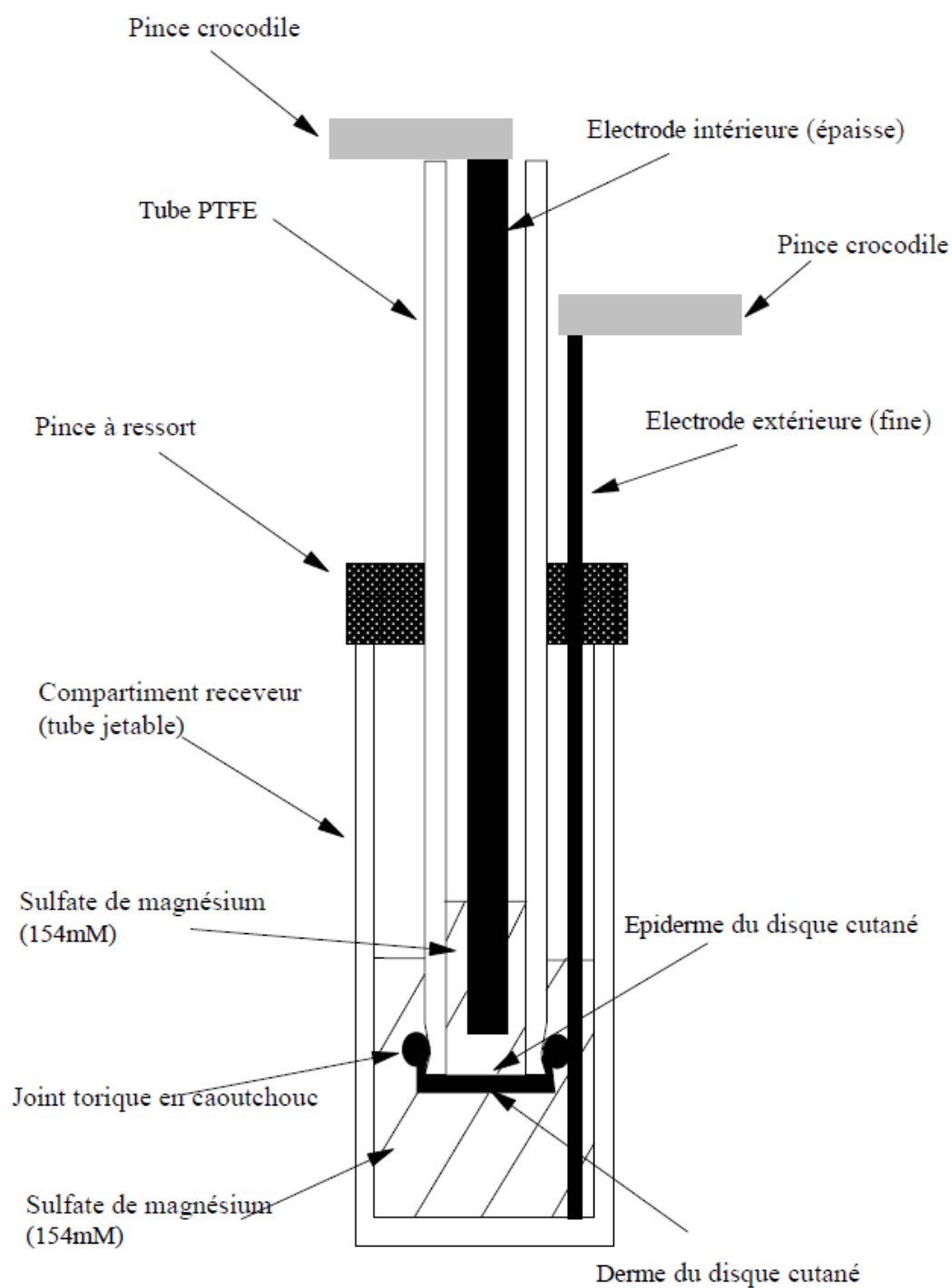
FIGURE1: APPAREIL POUR L'ESSAI DE RET SUR PEAU DE RAT
