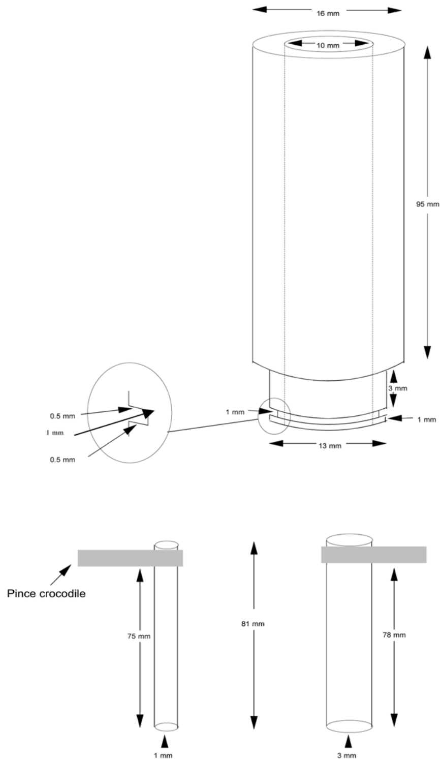
FIGURE2: DIMENSIONS DU TUBE PTFE (POLYTETRAFLUOROETHYLENE), DES TUBES RECEVEURS ET DES ELECTRODES UTILISES
