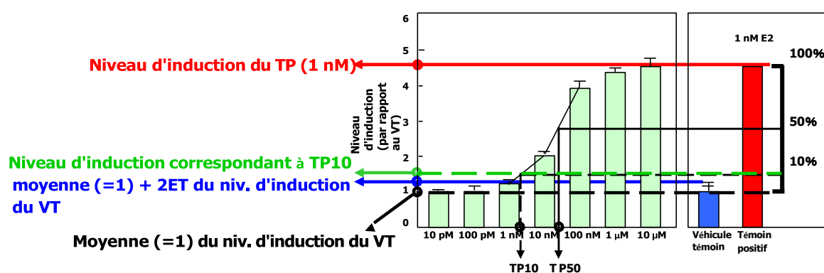
Figure 1. Exemple de déduction des valeurs relatives au TP. Le TP (1 nM de E2) est inclus dans chaque plaque d'essai
