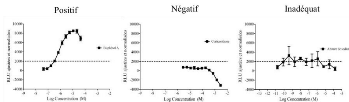
Graphique 5: Exemples de résultats positifs, négatifs et inadéquats pour l'effet agoniste
