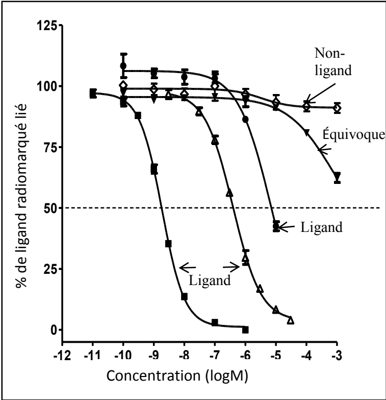
Graphique 1. Exemples de classification d'un produit chimique d'essai grâce à la courbe de liaison compétitive.
