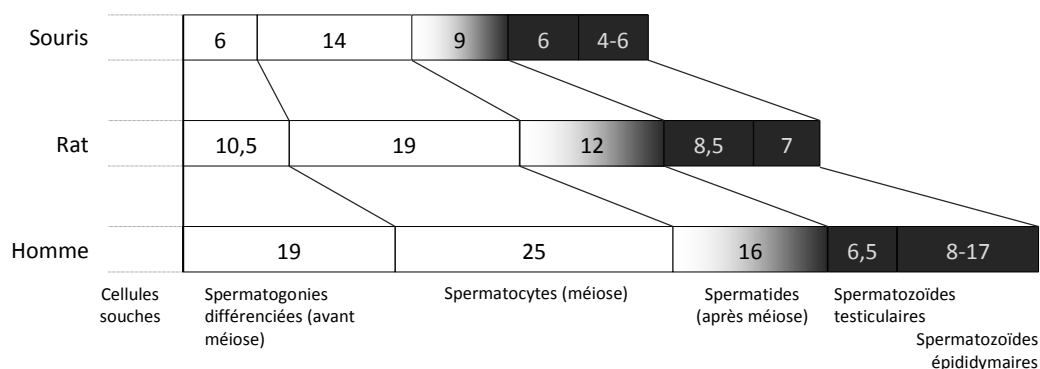
Fig.1: Comparaison de la durée (en jours) du développement des cellules germinales mâles chez la souris, le rat et l'homme. La réparation de l'ADN ne se produit pas pendant les périodes indiquées en grisé.
