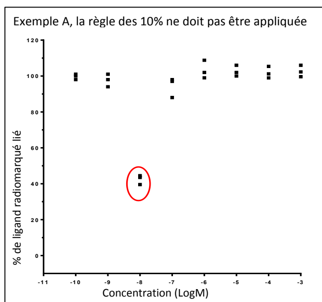
Graphique 3: Exemples de courbes de liaison compétitive dans lesquelles il ne faut pas appliquer la règle des 10 %.
