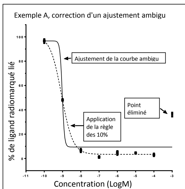
Graphique 2: Exemples de courbes de liaison compétitive avec ou sans application de la règle des 10 %.
