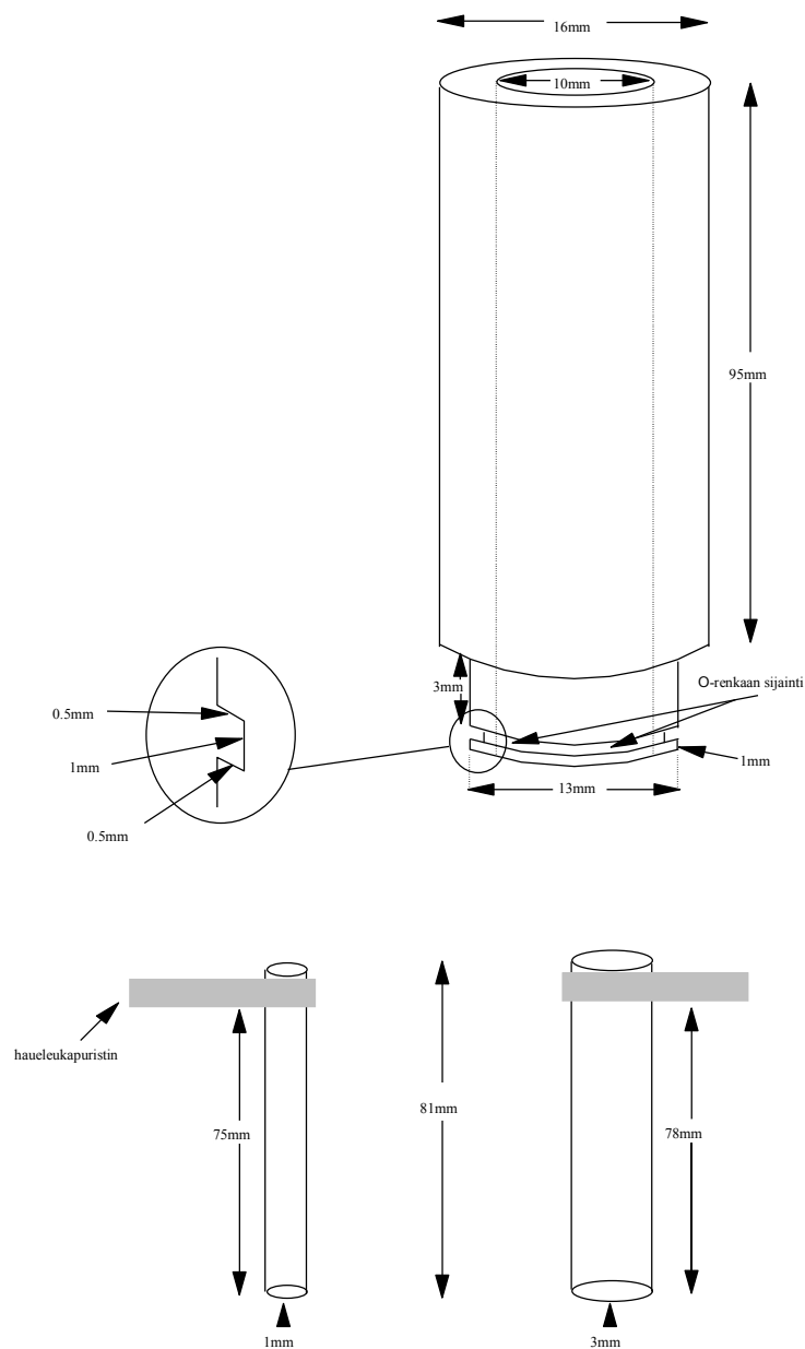
KUVA 2: POLYTETRAFLUOROETYLEENIPUTKEN (PTFE-PUTKEN), KOEASTIOIDEN JA ELEKTRODIEN MITAT
