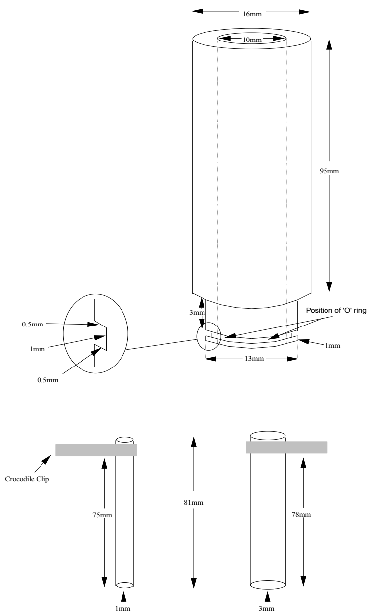
ΣΧΗΜΑ 2: ΔΙΑΣΤΑΣΕΙΣ ΤΟΥ ΣΩΛΗΝΑ ΠΟΛΥΤΕΤΡΑΦΘΟΡΟΑΙΘΥΛΕΝΙΟΥ (PTFE), ΤΟΥ ΥΠΟΔΟΧΕΑ ΚΑΙ ΤΩΝ ΗΛΕΚΤΡΟΔΙΩΝ ΠΟΥ ΧΡΗΣΙΜΟΠΟΙΗΘΗΚΑΝ
