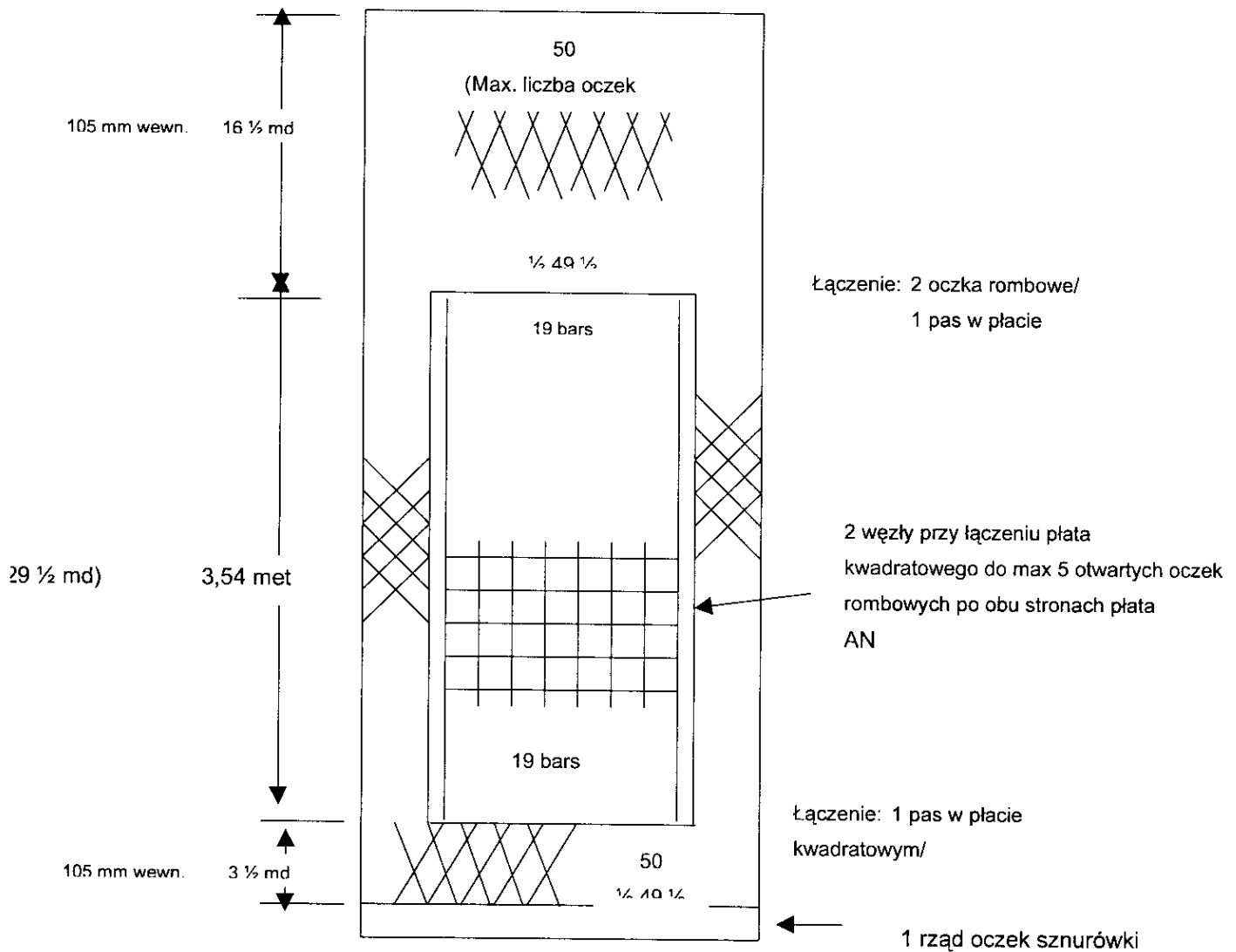
Rysunek 4c Konstrukcja górnego płatu w przypadku zachowania 20% rombownych oczek w górnym płacie i jednakowego rozdzielenia po obu stronach okna.
