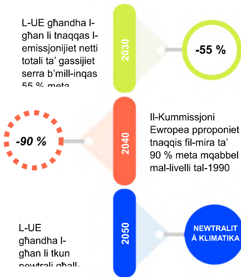
Illustrazzjoni 4: Miri klimatiċi ewlenin tal-UE
