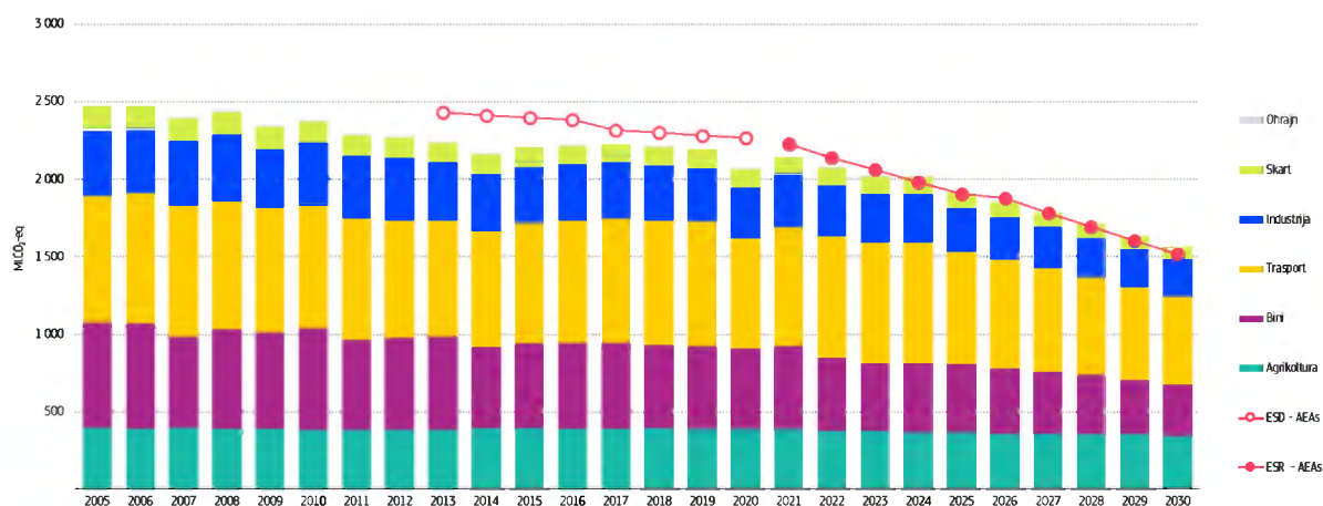
Illustrazzjoni 12: L-emissjonijiet fis-setturi koperti mil-leġiżlazzjoni dwar il-kondiviżjoni tal-isforzi 2005-2030 u l-allokazzjonijiet ta' emissjonijiet annwali, EU-27
