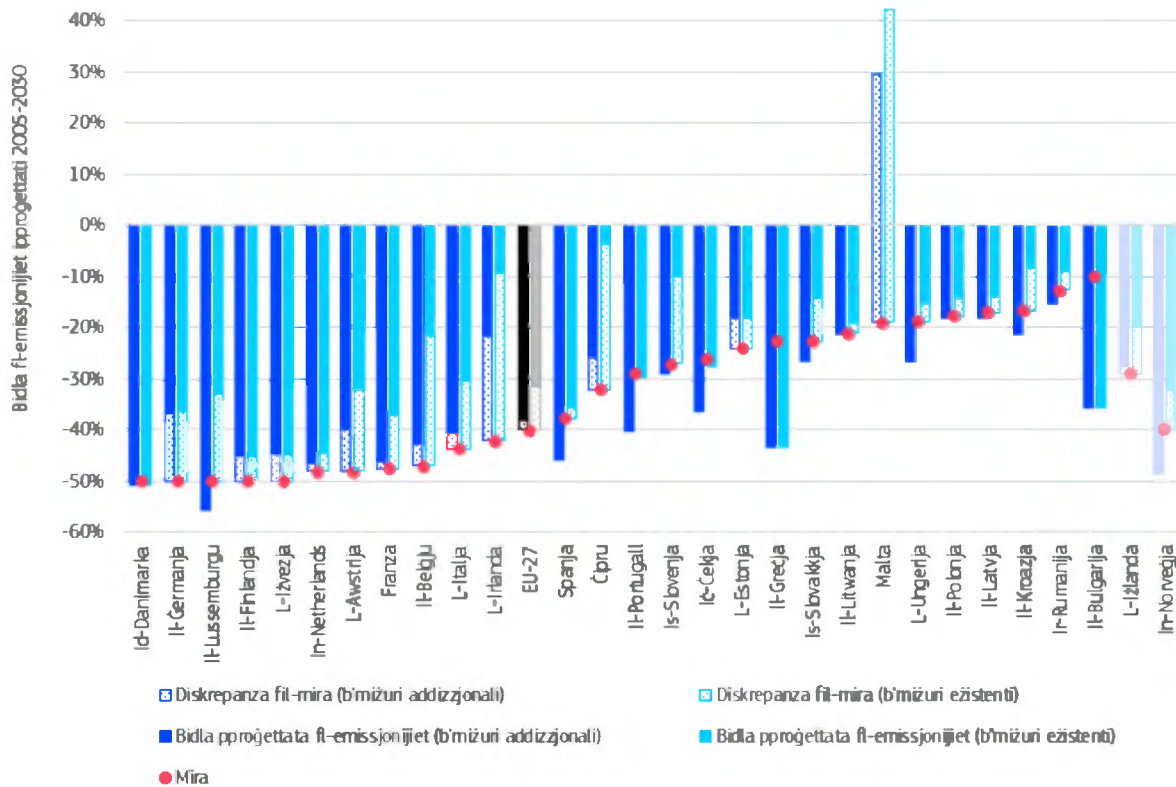
Illustrazzjoni 13: Bidla pproġettata tal-emissjonijiet tal-ESR u diskrepanza sal-mira fl-2030 (%)
