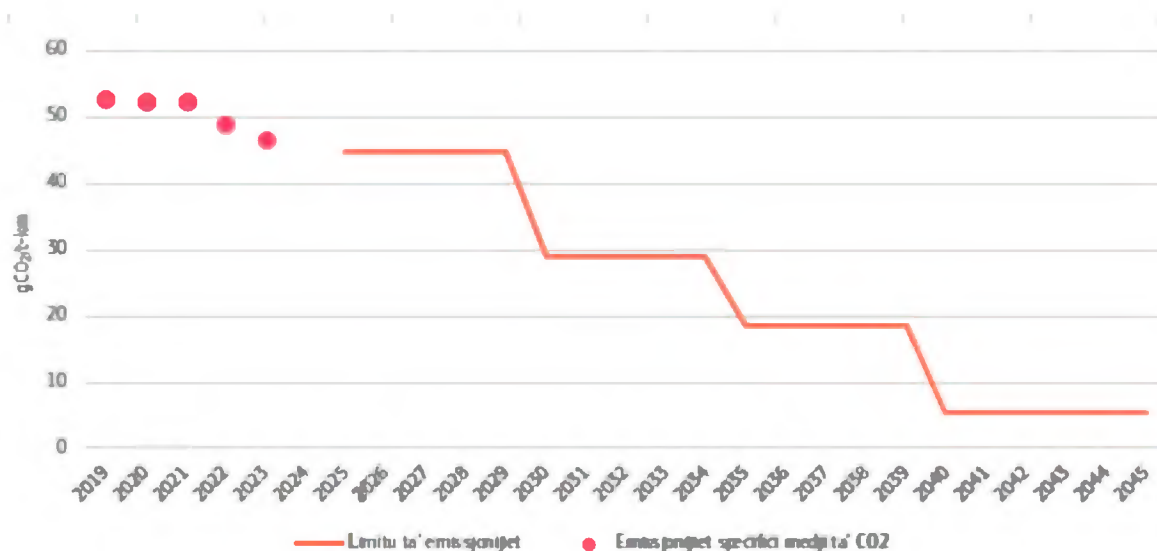
Illustrazzjoni 18: Emissjonijiet speċifiċi medji ta' CO 2 (tikek) u miri għall-flotta kollha tal-UE (linji) għal vetturi heavy-duty ġodda tal-gruppi ta' vetturi inizjalment regolati
