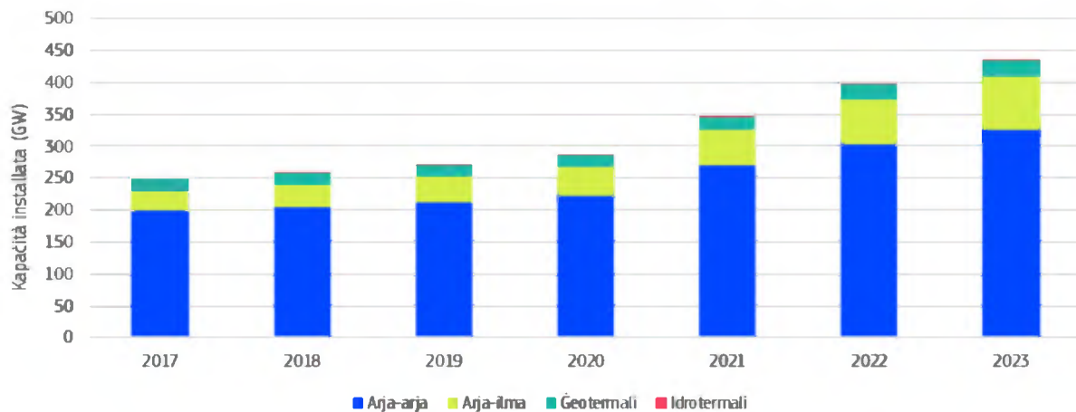
Illustrazzjoni 25: Kapaċità installata tal-pompi tas-sħana
