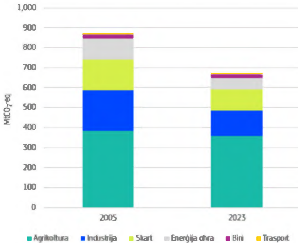
Illustrazzjoni 15: Emissjonijiet mhux tas-CO 2 skont l-ESR fl-2005 u fl-2023, skont is-settur
