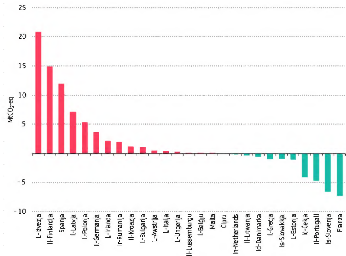
Illustrazzjoni 20: Diskrepanza pproġettata sal-miri nazzjonali tal-2030 b'miżuri addizzjonali, abbażi tal-projezzjonijiet tal-Istati Membri għall-2030 (MtCO 2 -eq)
