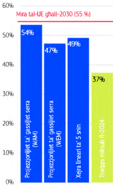
Illustrazzjoni 6: Tnaqqis ipproġettat fl-emissjonijiet fil-perjodu 1990–2030 u diskrepanza sal-mira skont il-politiki ewlenin
