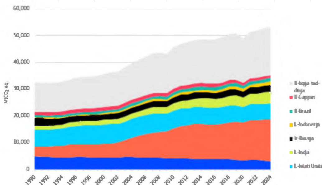
Illustrazzjoni 3: Emissjonijiet globali ta' gassijiet serra (1990-2024)
