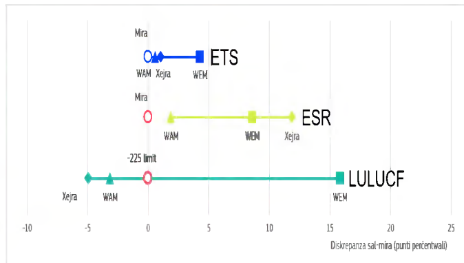
Illustrazzjoni 6: Tnaqqis ipproġettat fl-emissjonijiet fil-perjodu 1990–2030 u diskrepanza sal-mira skont il-politiki ewlenin
