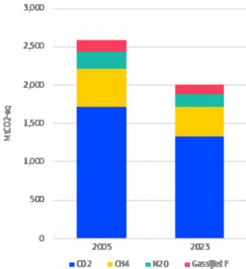
Illustrazzjoni 14: Emissjonijiet skont l-ESR fl-2005 u fl-2023, skont it-tip ta' gass
