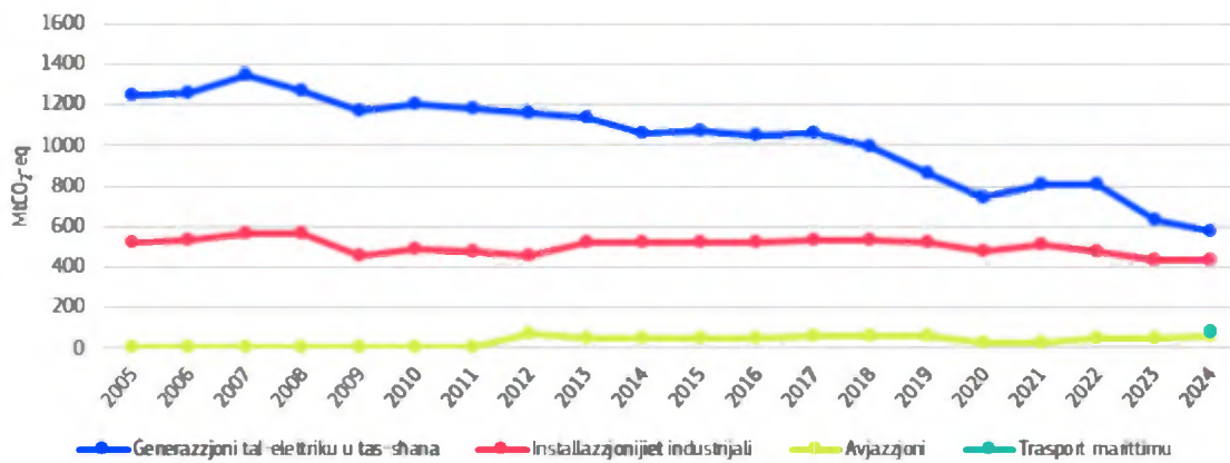
Illustrazzjoni 10: Emissjonijiet taht l-EU ETS fl-UE skont is-settur
