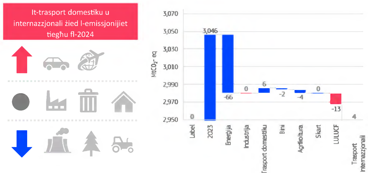
Illustrazzjoni 2: Bidla fl-emissjonijiet ta' gassijiet serra tal-UE fl-2024 skont is-settur
