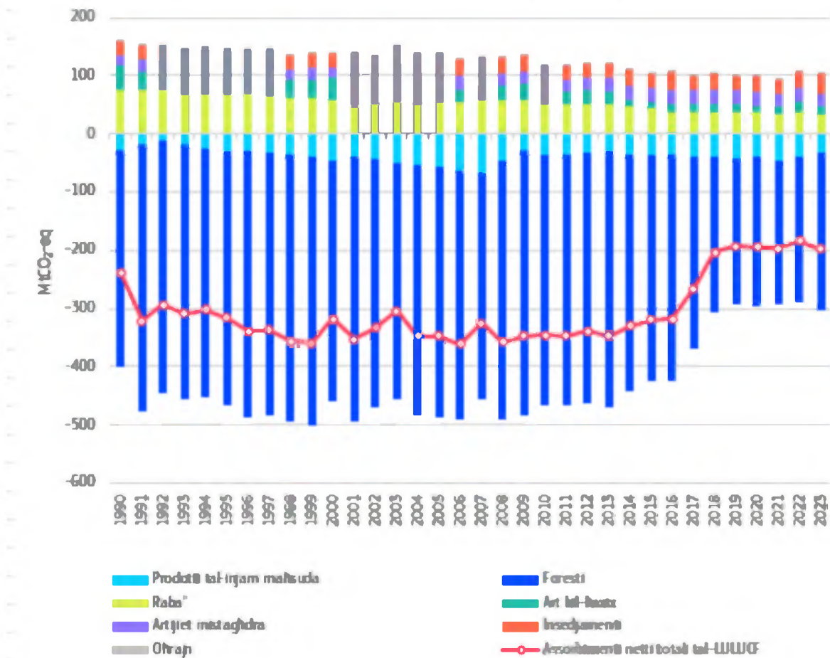
Illustrazzjoni 19: Emissjonijiet u assorbimenti tas-settur tal-art fil-perjodu 1990-2023 skont il-kategorija ewlenija tal-użu tal-art (EU-27)
