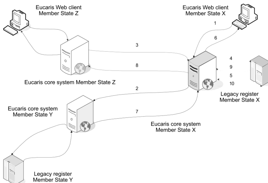
Slika 5: Tipi sporočil za kontrolno beleženje
