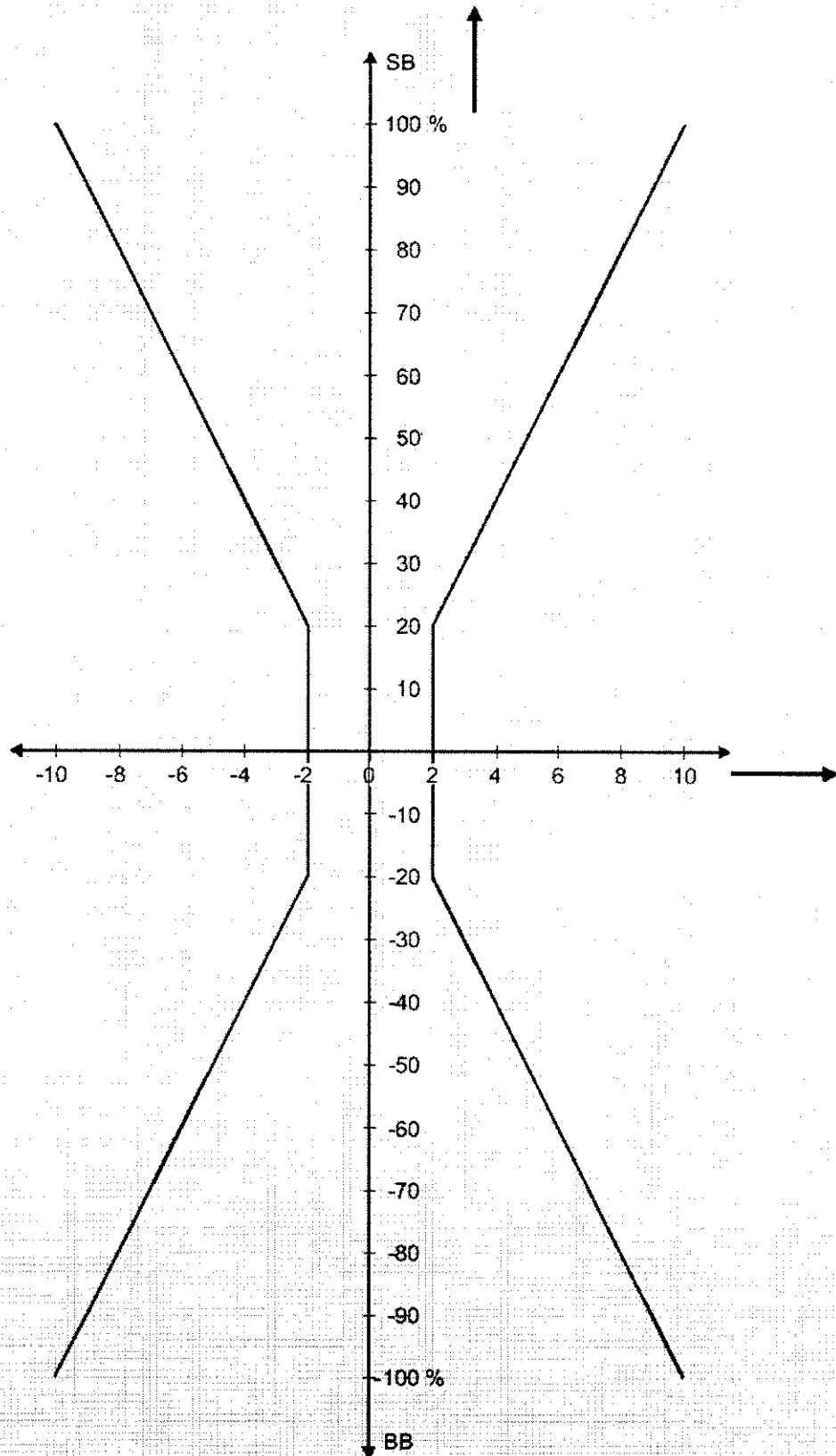
Figuur 1: Tolerantiegrenzen voor bochtenwijzers
