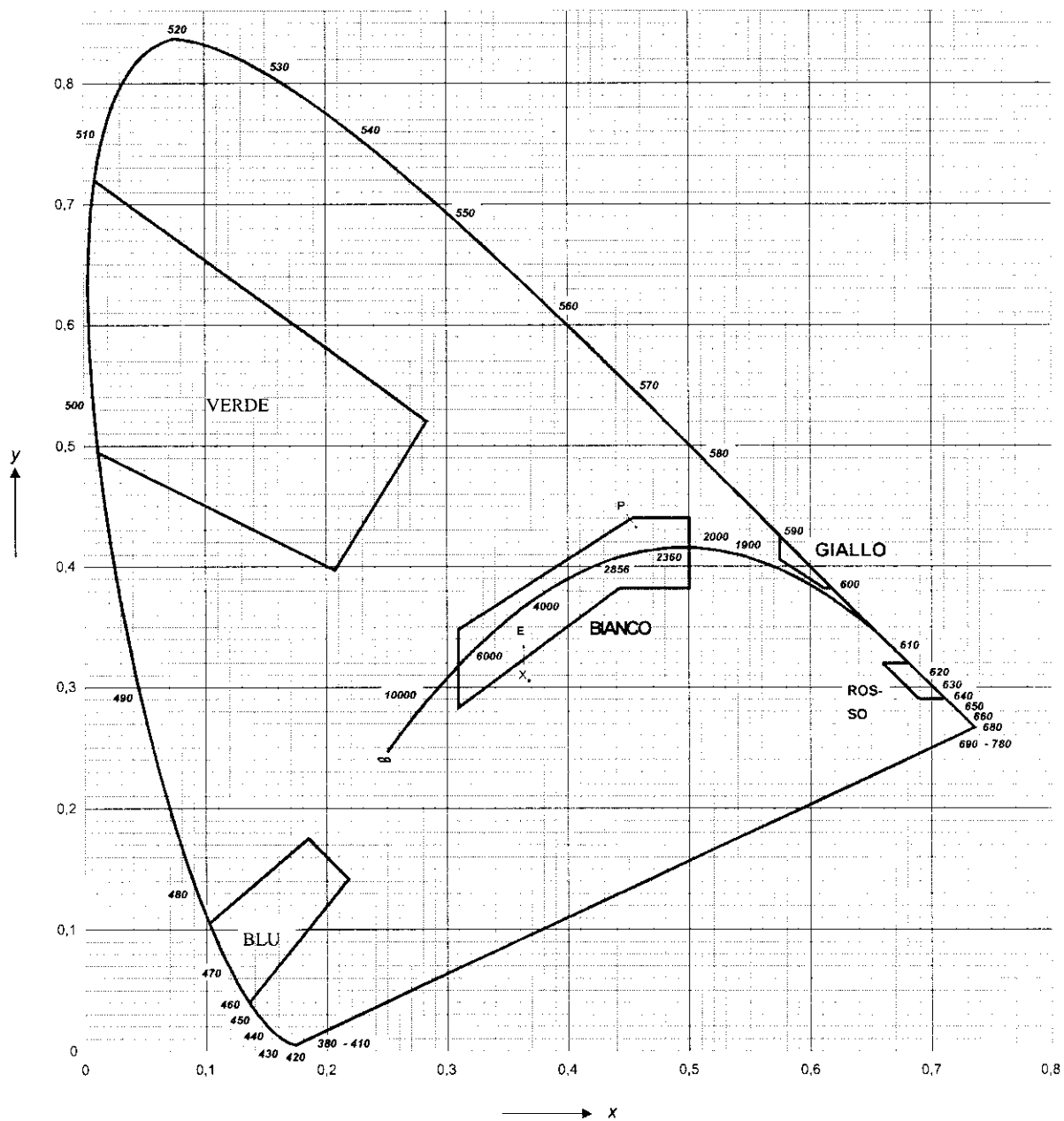
Diagramma colorimetrico IEC
