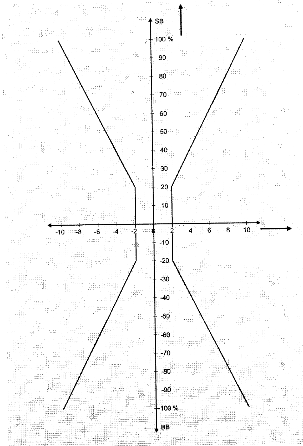
Figuur 1: Tolerantiegrenzen voor bochtaanwijzers
