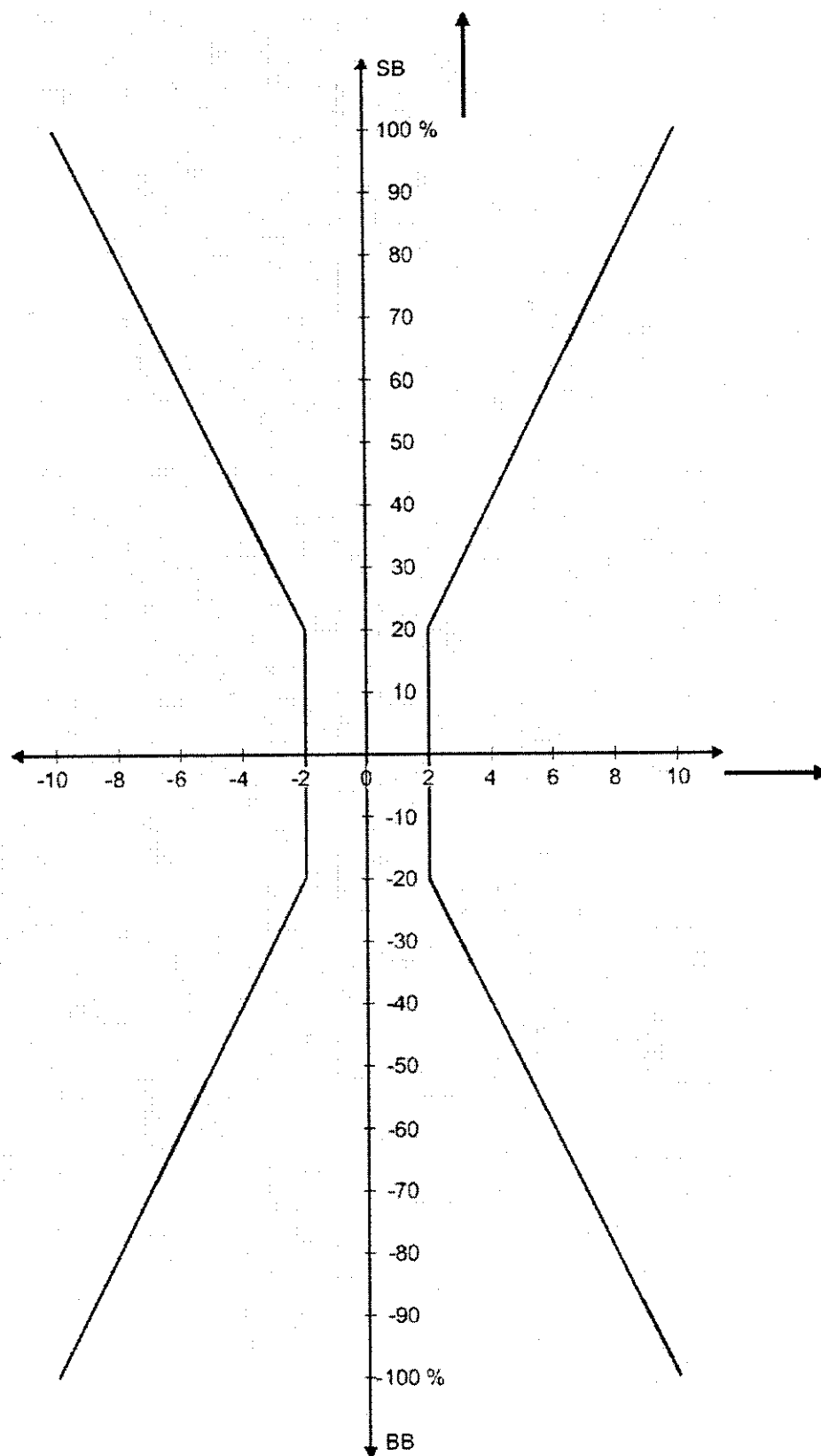
Figura 1: Tolleranze di errore per gli indicatori della velocità di accostata
