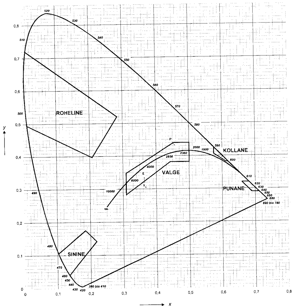
IEC värvusdiagramm,
