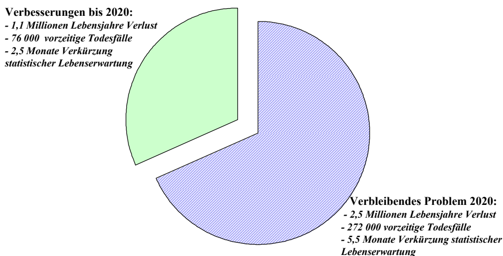
Abb. 2: Auswirkung von Partikeln auf die Sterblichkeit 2000 & 2020 (derzeitige Strategien)
