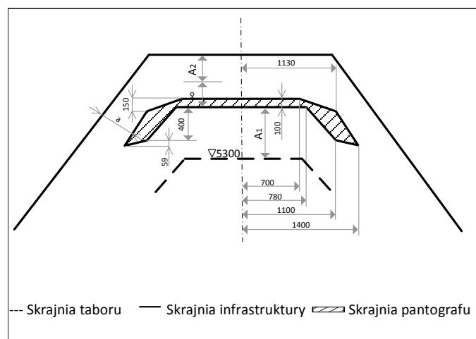
Rys. D.3 —Statyczna skrajnia pantografu dla systemu o szerokości torów 1520mm
