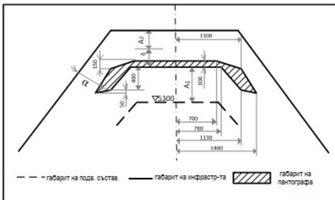
Фигура Г.3 — Статичен габарит на пантографа за система с междурелсие 1520 mm
