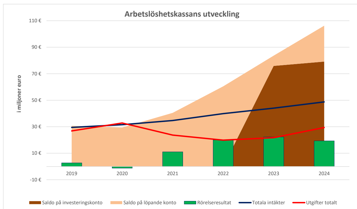
Fig. 3.3.1 Arbetslöshetskassans utveckling
