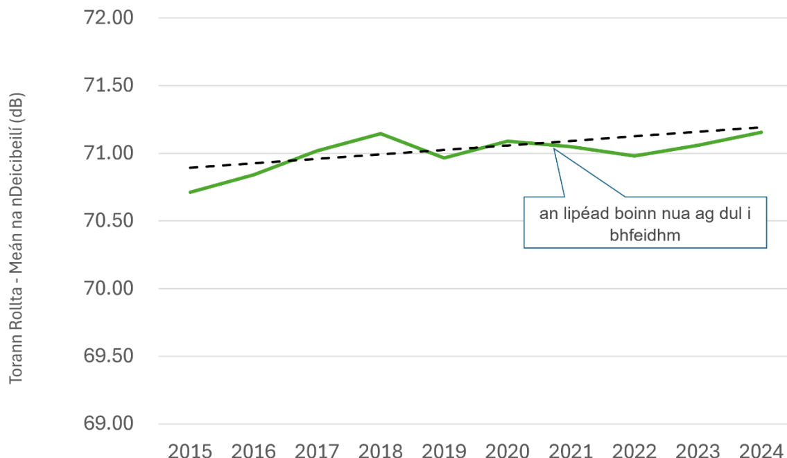
Fíor 6: Torann seachtrach rollta bhoinn C1.
