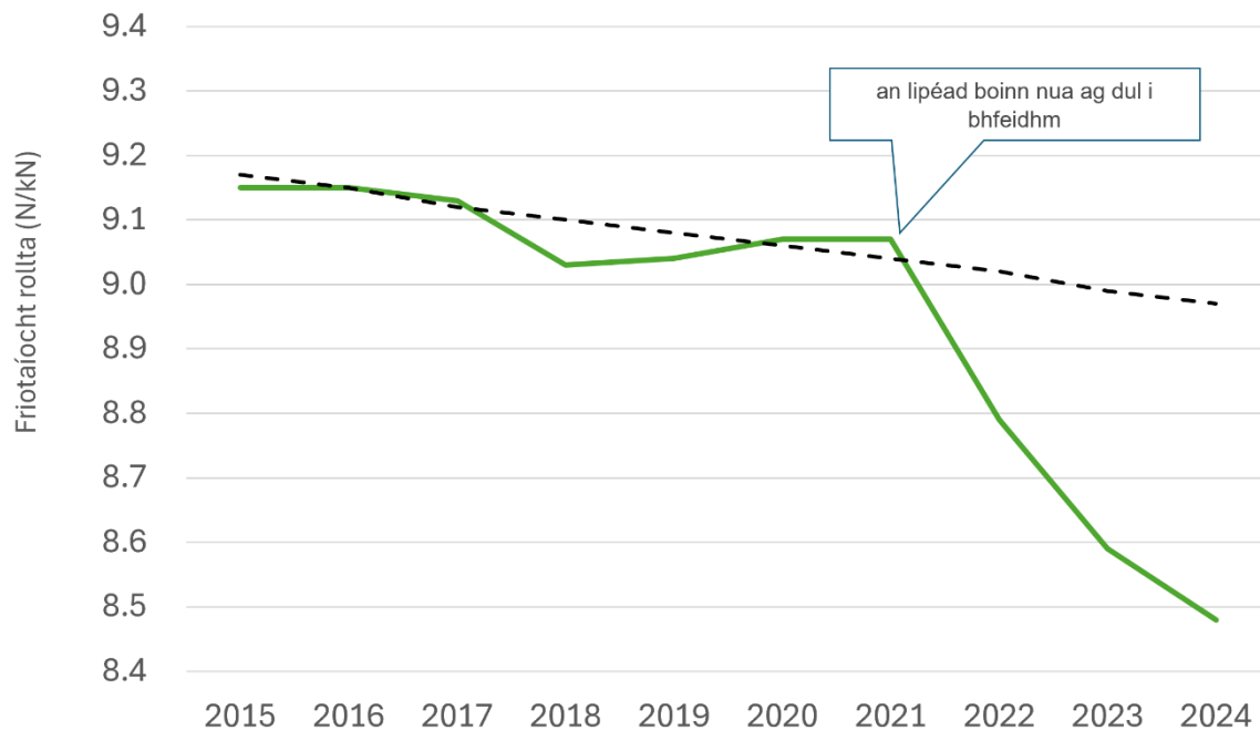
Fíor 4: Friotaíocht rollta bhonn C1.
