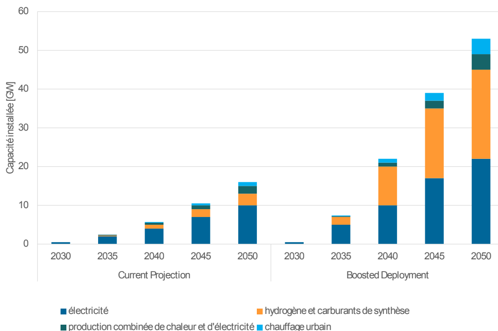
Figure 5 – Scénarios de déploiement (actuel à gauche, renforcé à droite) des PRM avec parts de l’approvisionnement en chaleur/hydrogène (current projection : projection actuelle boosted deployment : déploiement renforcé)
