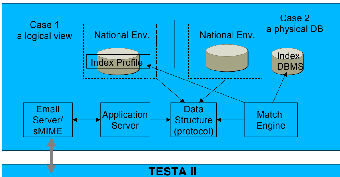
Fig. Topoloġija ġenerali ta' l-applikazzjoni
