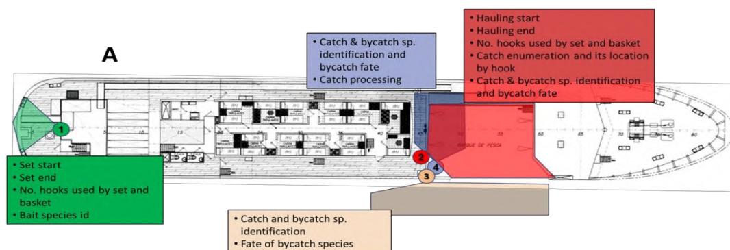
FIGURA 1. Configurazione delle telecamere e attività di pesca da registrare sul ponte principale (A) e sul ponte dei pozzi (B) di una tonniere con rete a circuizione di classe 6 e di un peschereccio di classe 2 (C).
