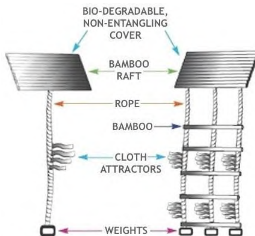
Figur: Eksempel på en bionedbrydelig FAD, der ikke resulterer i indfiltring
