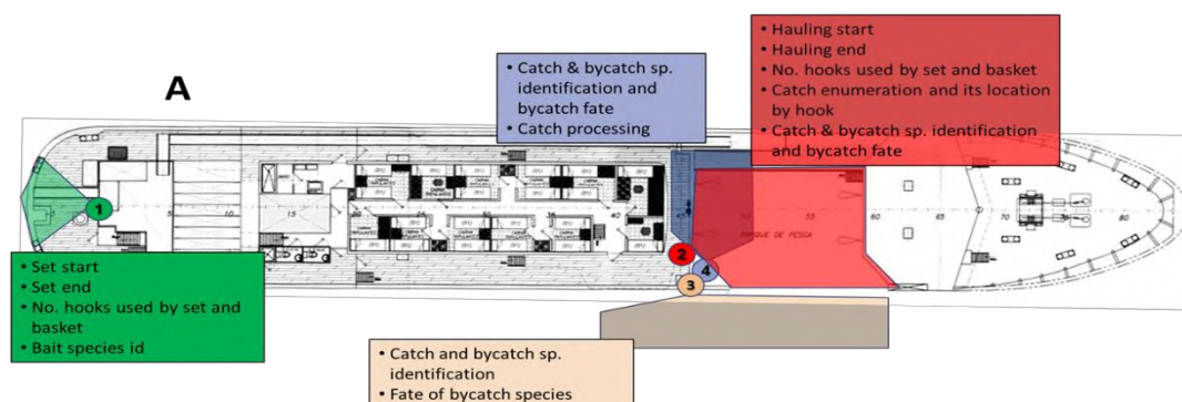
FIGUR 1 Kamerakonfiguration og de fiskeriaktiviteter, der skal optages på hoveddækket (A) og tankdækket (B) på notfartøjer til tunfiskeri i klasse 6 og på et fartøj i klasse 2 (C).
