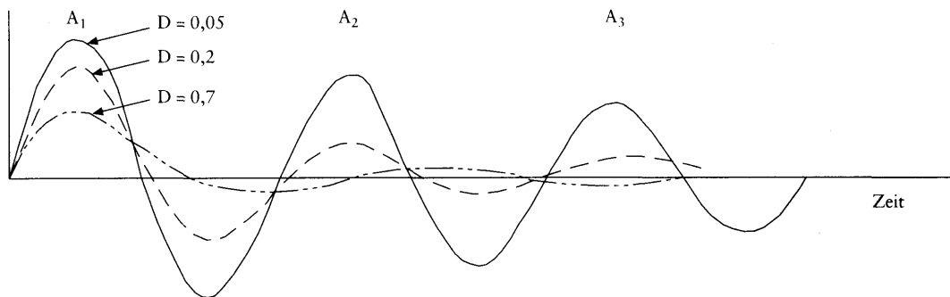
Abbildung 2 Gedämpfte Sinuskurve bei einer kurzzeitigen freien Schwingung
